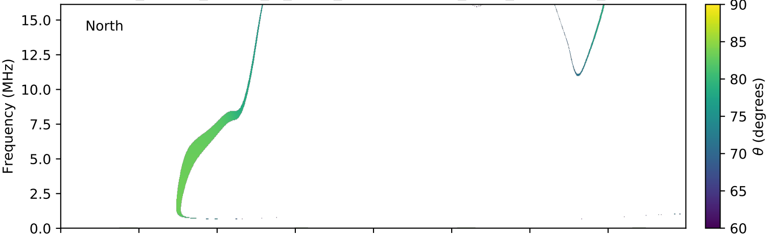
expres_cassini_jupiter_io_isaac_lossc-wid1deg_3kev_20020501_v01.cdf
