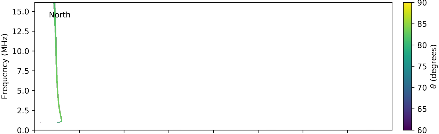
expres_cassini_jupiter_io_isaac_lossc-wid1deg_3kev_20020301_v01.cdf
