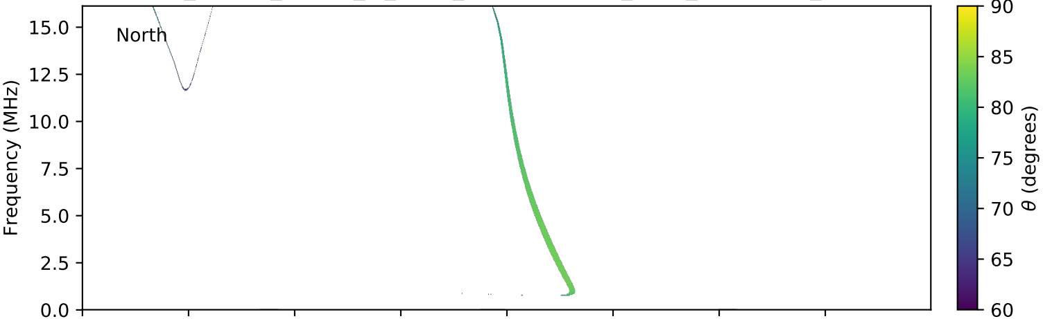
expres_cassini_jupiter_io_isaac_lossc-wid1deg_3kev_20020117_v01.cdf
