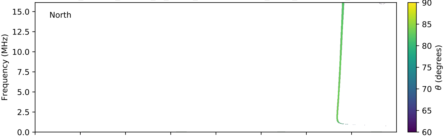
expres_cassini_jupiter_io_isaac_lossc-wid1deg_3kev_20020116_v01.cdf
