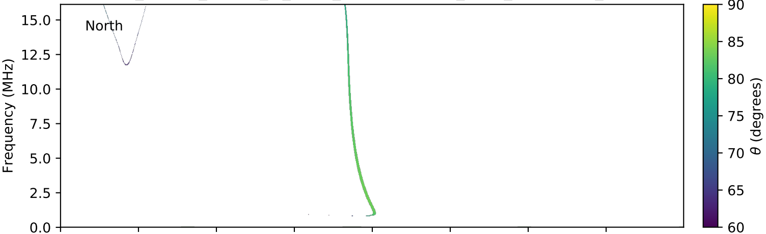
expres_cassini_jupiter_io_isaac_lossc-wid1deg_3kev_20020110_v01.cdf
