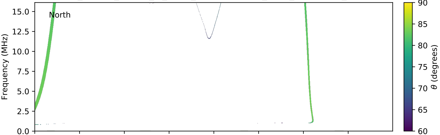
expres_cassini_jupiter_io_isaac_lossc-wid1deg_3kev_20020108_v01.cdf
