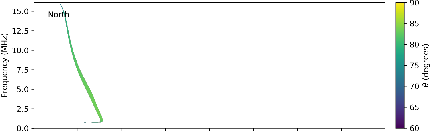
expres_cassini_jupiter_io_isaac_lossc-wid1deg_3kev_20020105_v01.cdf
