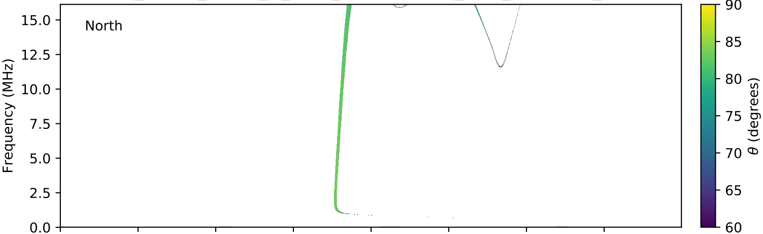
expres_cassini_jupiter_io_isaac_lossc-wid1deg_3kev_20020104_v01.cdf
