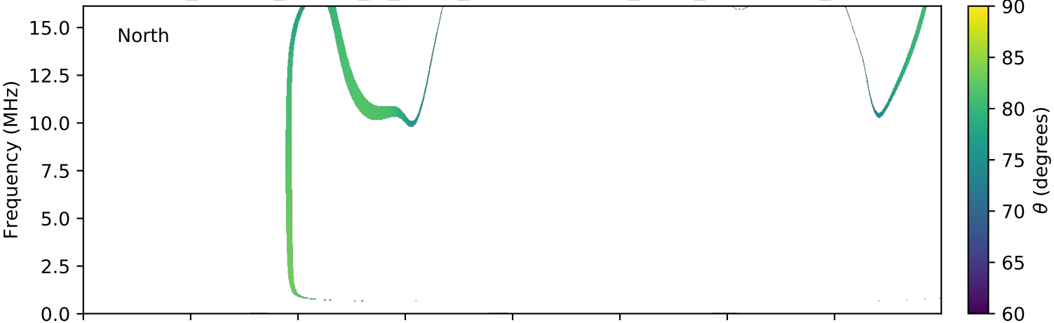
expres_cassini_jupiter_io_isaac_lossc-wid1deg_3kev_20010920_v01.cdf
