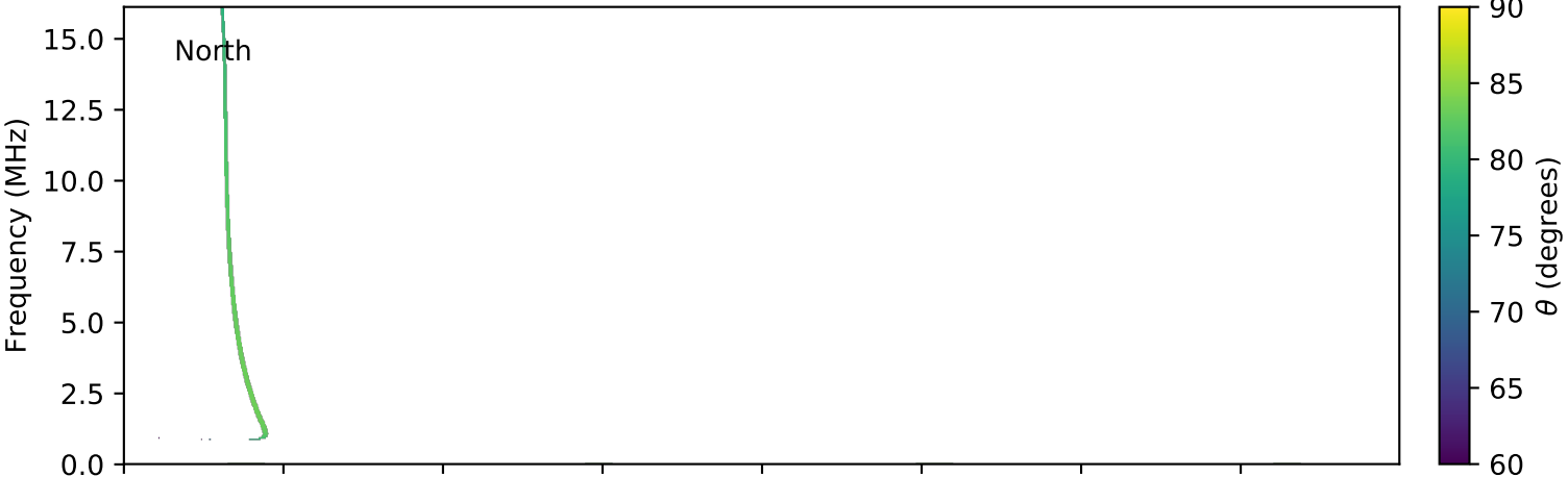
expres_cassini_jupiter_io_isaac_lossc-wid1deg_3kev_20010905_v01.cdf
