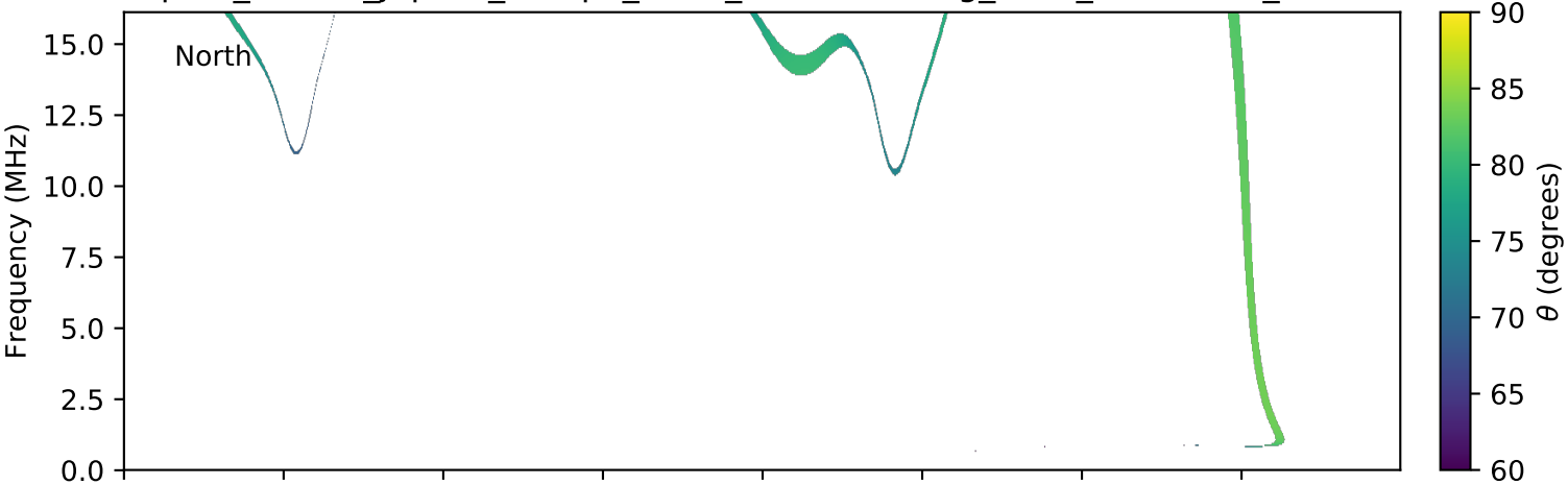
expres_cassini_jupiter_europa_isaac_lossc-wid1deg_3kev_20010905_v01.cdf
