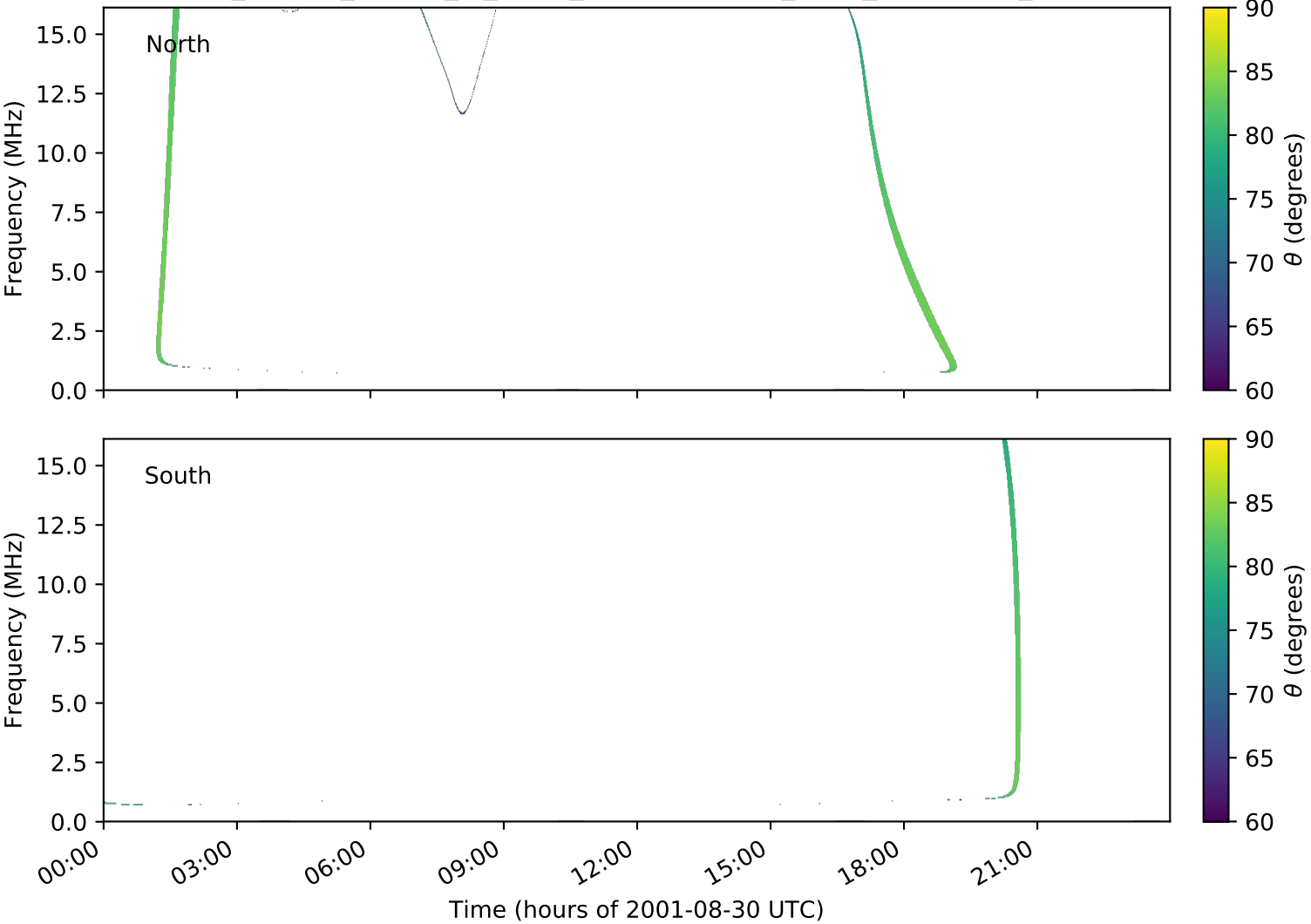
expres_cassini_jupiter_io_isaac_lossc-wid1deg_3kev_20010830_v01.cdf
