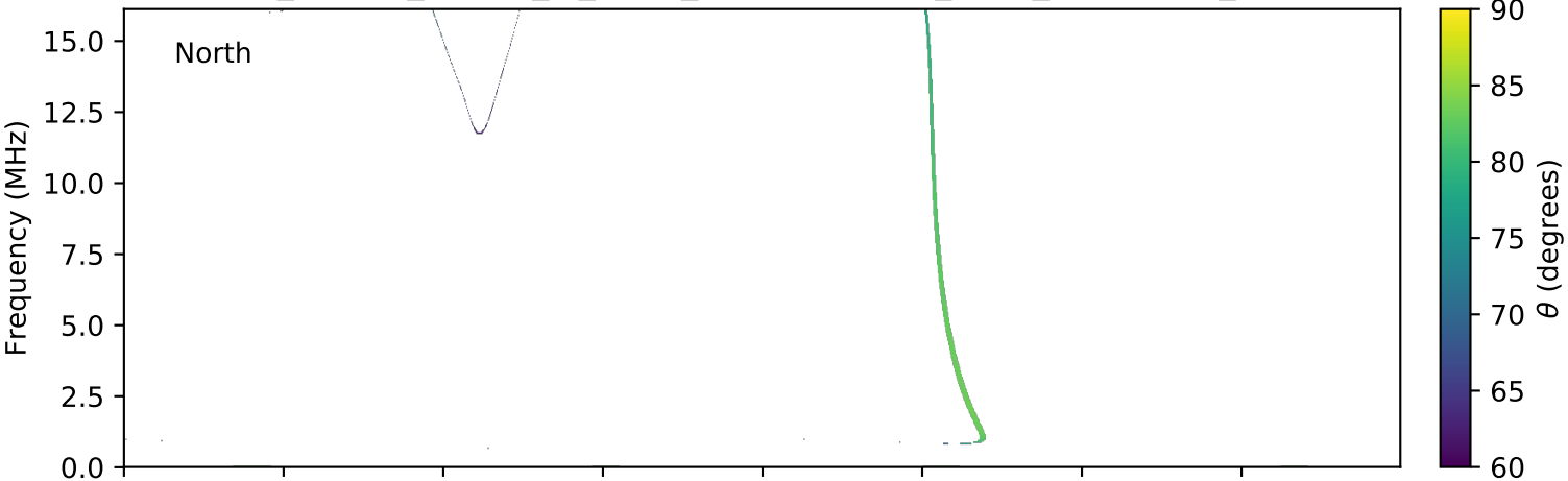
expres_cassini_jupiter_io_isaac_lossc-wid1deg_3kev_20010220_v01.cdf
