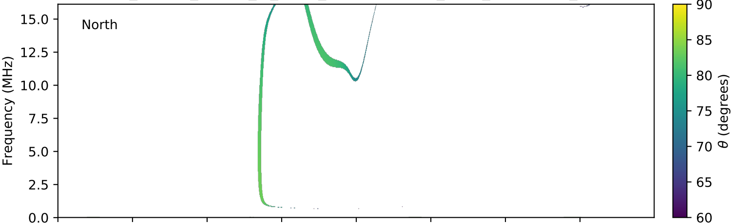
expres_cassini_jupiter_io_isaac_lossc-wid1deg_3kev_20010216_v01.cdf
