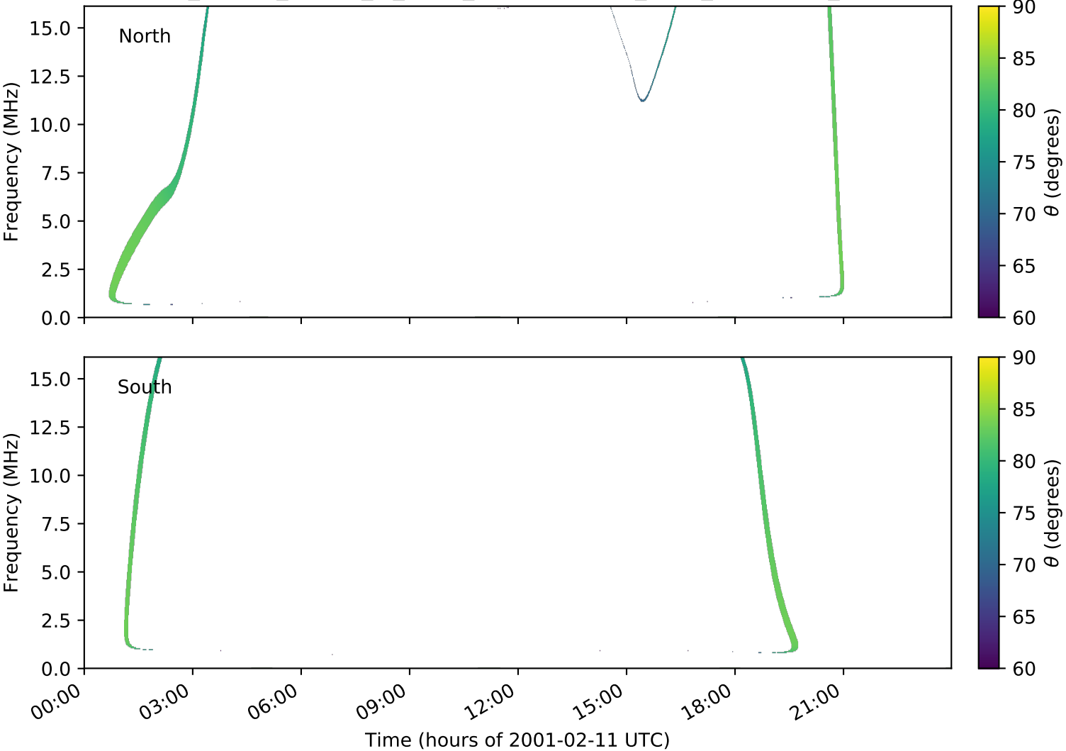
expres_cassini_jupiter_io_isaac_lossc-wid1deg_3kev_20010211_v01.cdf
