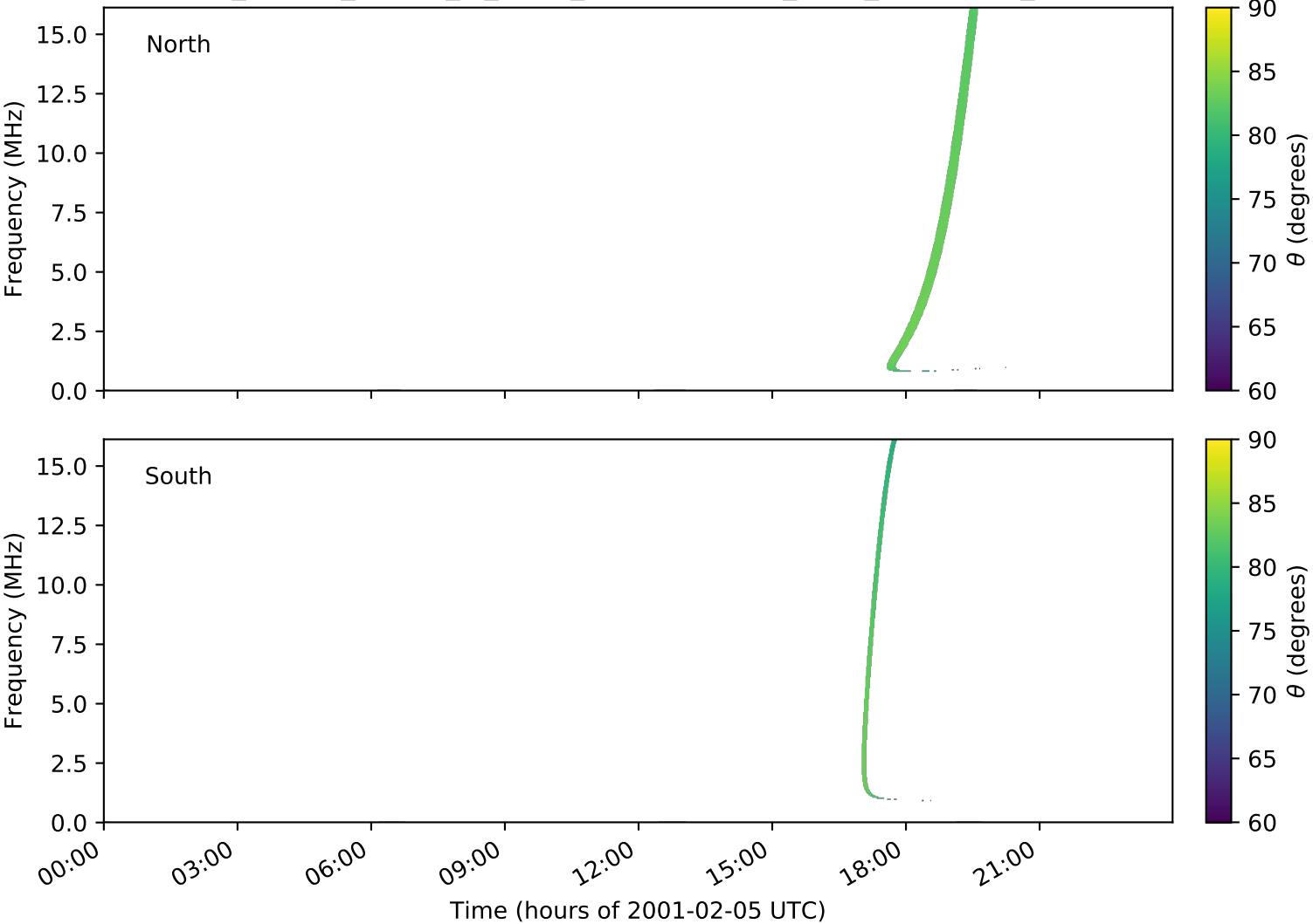
expres_cassini_jupiter_io_isaac_lossc-wid1deg_3kev_20010205_v01.cdf
