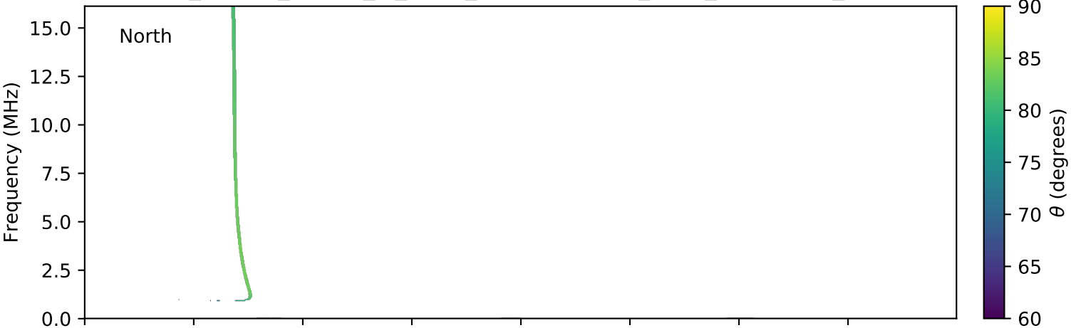
expres_cassini_jupiter_io_isaac_lossc-wid1deg_3kev_20010201_v01.cdf
