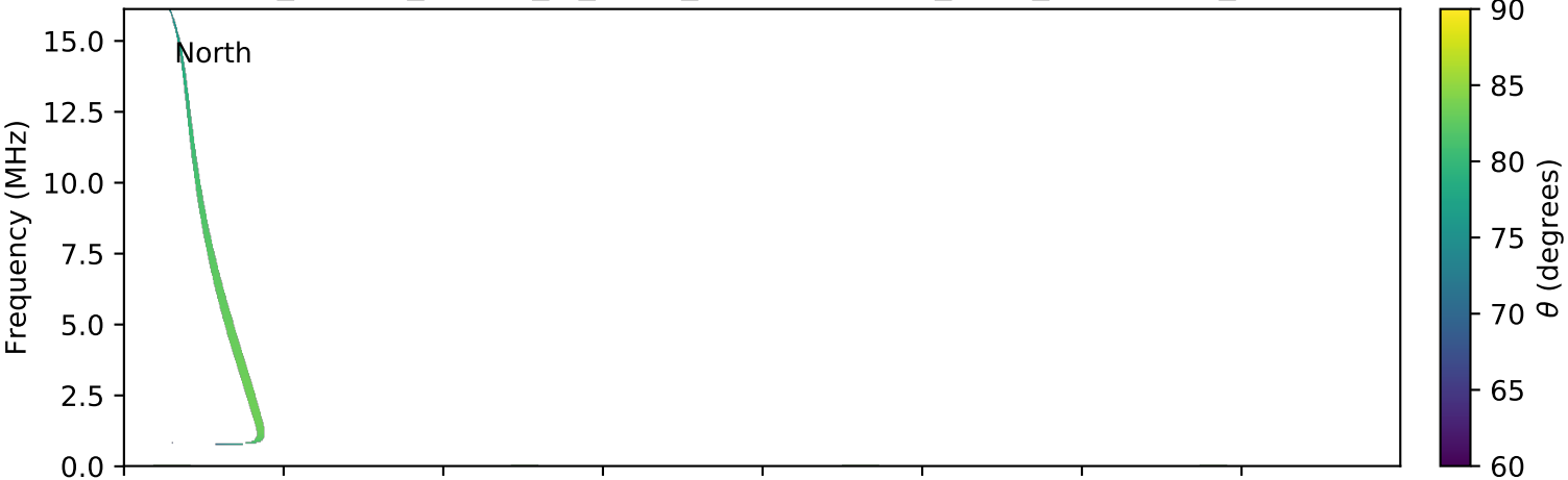
expres_cassini_jupiter_io_isaac_lossc-wid1deg_3kev_20001220_v01.cdf
