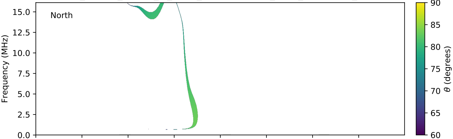
expres_cassini_jupiter_io_isaac_lossc-wid1deg_3kev_20001209_v01.cdf
