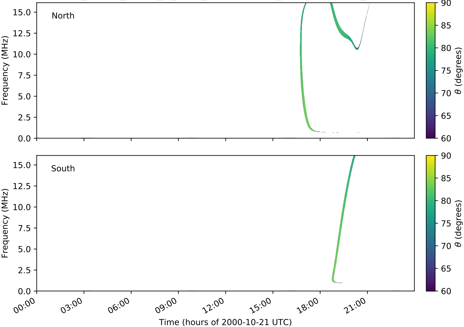
expres_cassini_jupiter_io_isaac_lossc-wid1deg_3kev_20001021_v01.cdf
