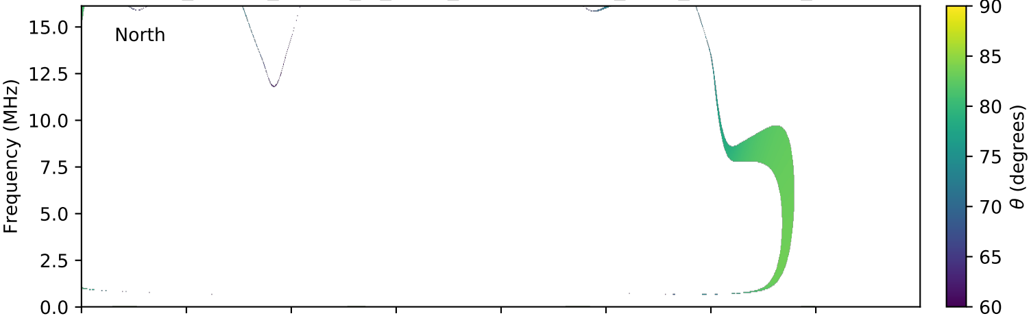
expres_cassini_jupiter_io_isaac_lossc-wid1deg_3kev_20001020_v01.cdf
