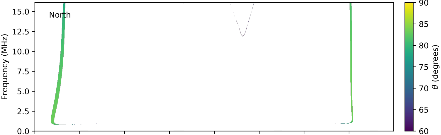
expres_cassini_jupiter_io_isaac_lossc-wid1deg_3kev_20001004_v01.cdf
