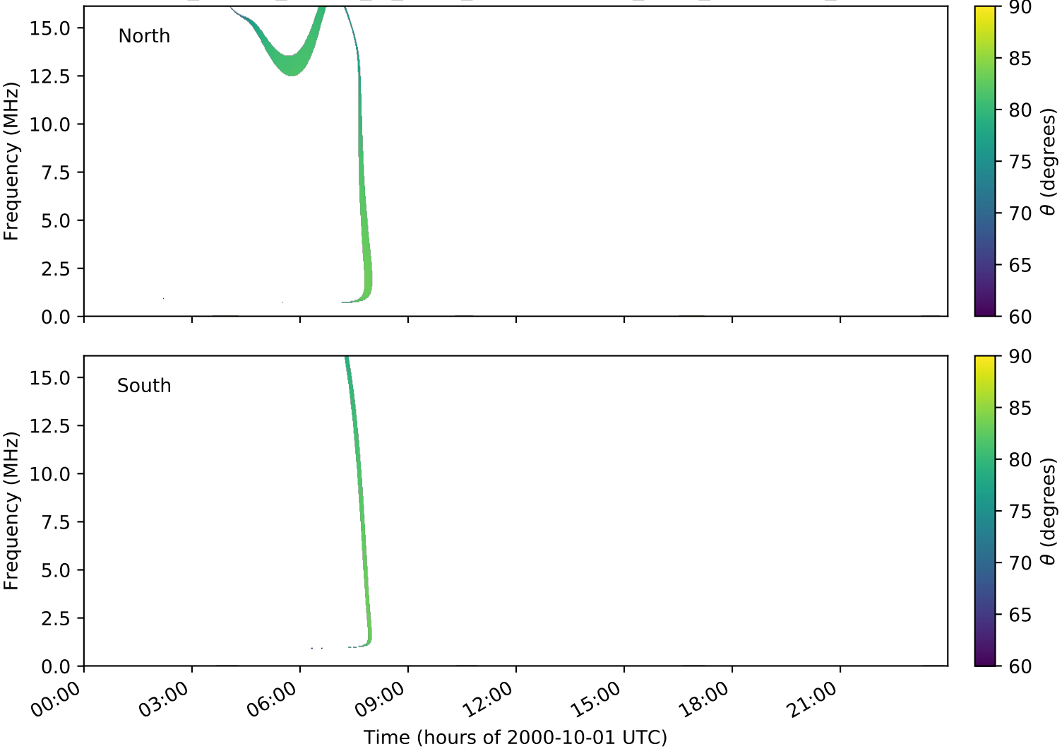
expres_cassini_jupiter_io_isaac_lossc-wid1deg_3kev_20001001_v01.cdf
