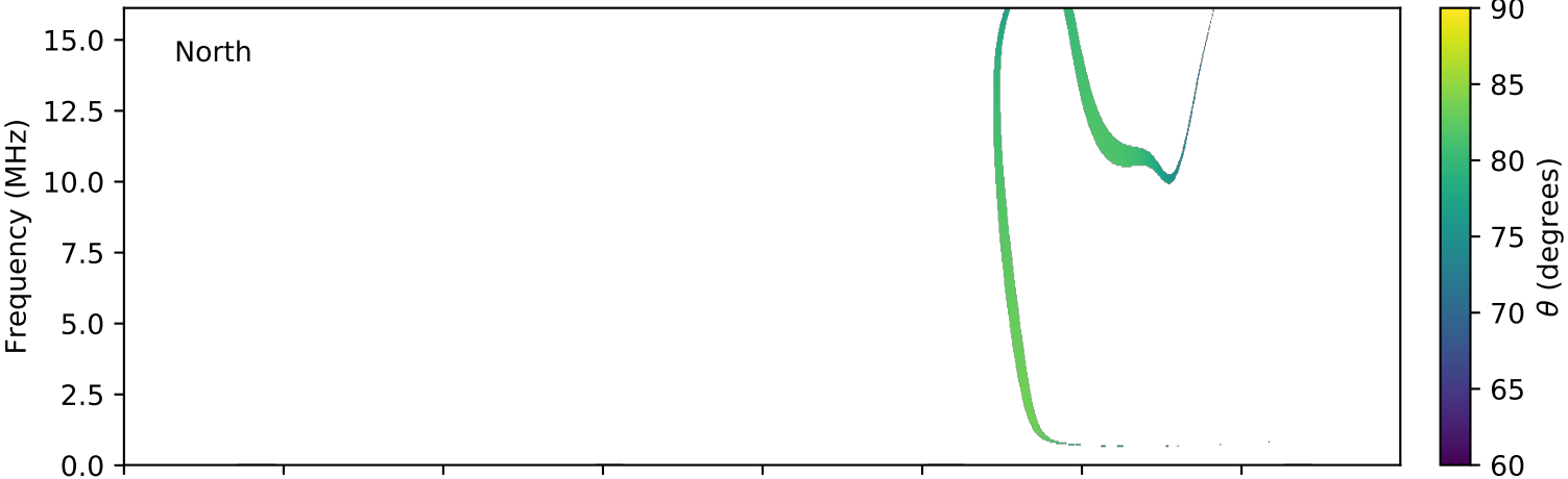
expres_cassini_jupiter_io_isaac_lossc-wid1deg_3kev_20000420_v01.cdf
