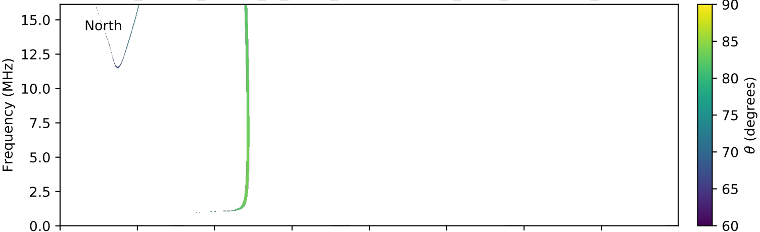
expres_cassini_jupiter_io_isaac_lossc-wid1deg_3kev_20000301_v01.cdf
