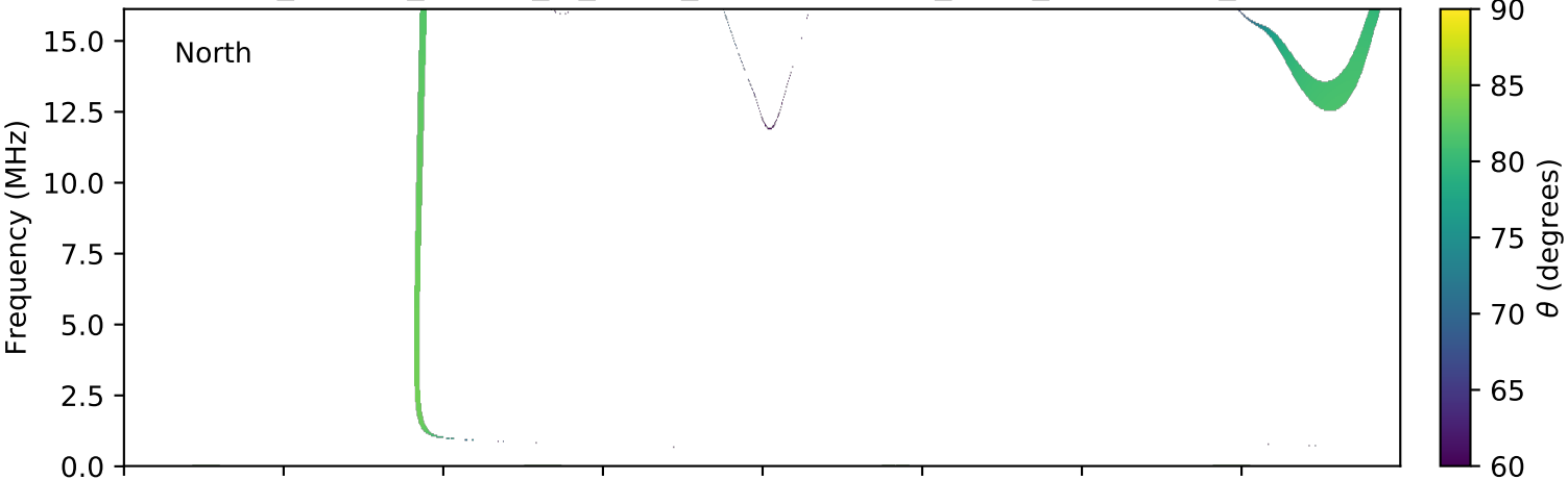
expres_cassini_jupiter_io_isaac_lossc-wid1deg_3kev_20000208_v01.cdf
