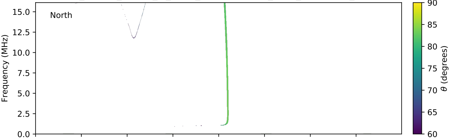
expres_cassini_jupiter_io_isaac_lossc-wid1deg_3kev_20000205_v01.cdf
