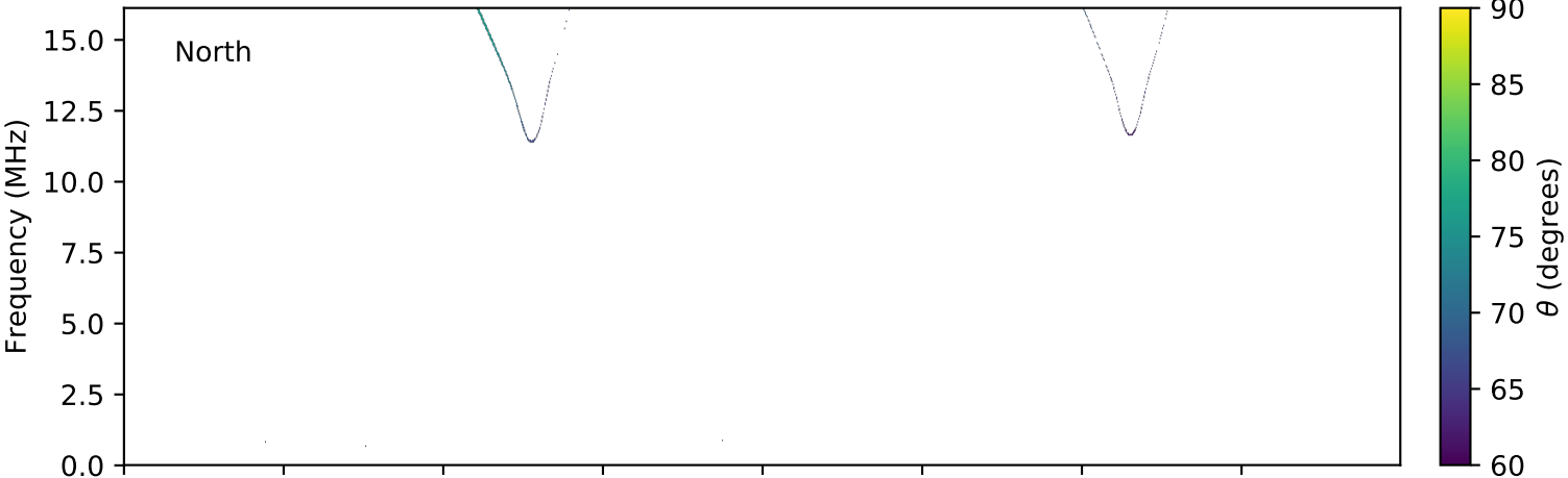
expres_cassini_jupiter_europa_isaac_lossc-wid1deg_3kev_20000209_v01.cdf
