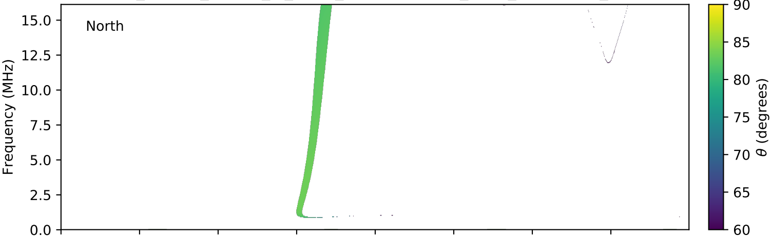
expres_cassini_jupiter_io_isaac_lossc-wid1deg_3kev_20000130_v01.cdf
